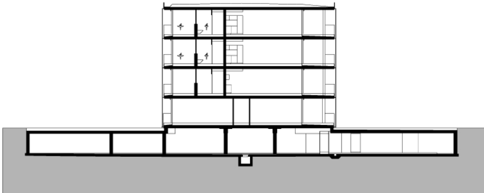
Querschnitt
